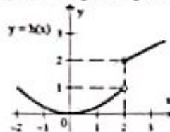
B f(x) e h(x)
