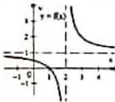
A f(x) e g(x)
