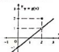
C h(x) D g(x)
